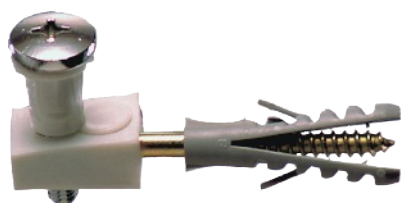
010 (MODELO LATERAL) Suministrado en bolsa de 2 unidades con fijación completa y taco nylon.
